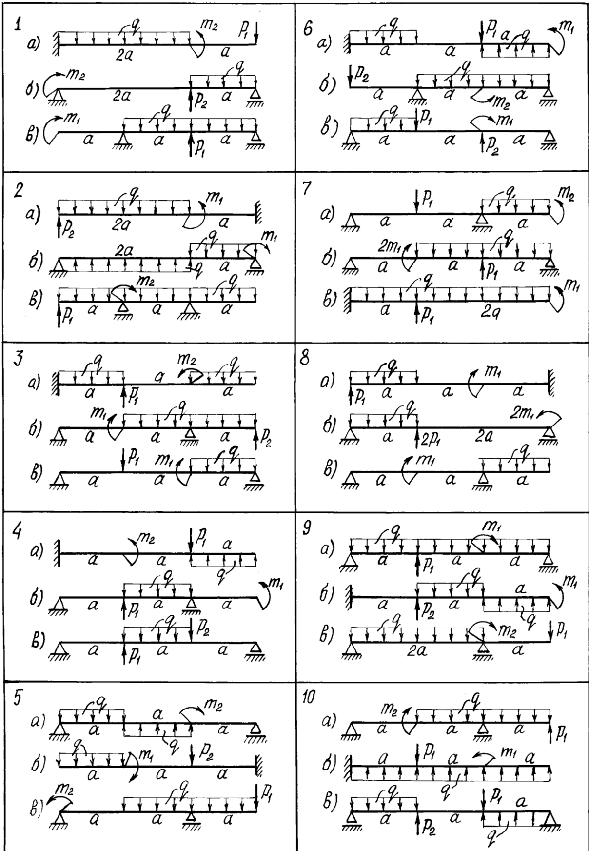
Рис. 13. Расчетные схемы балок к задаче № 5
